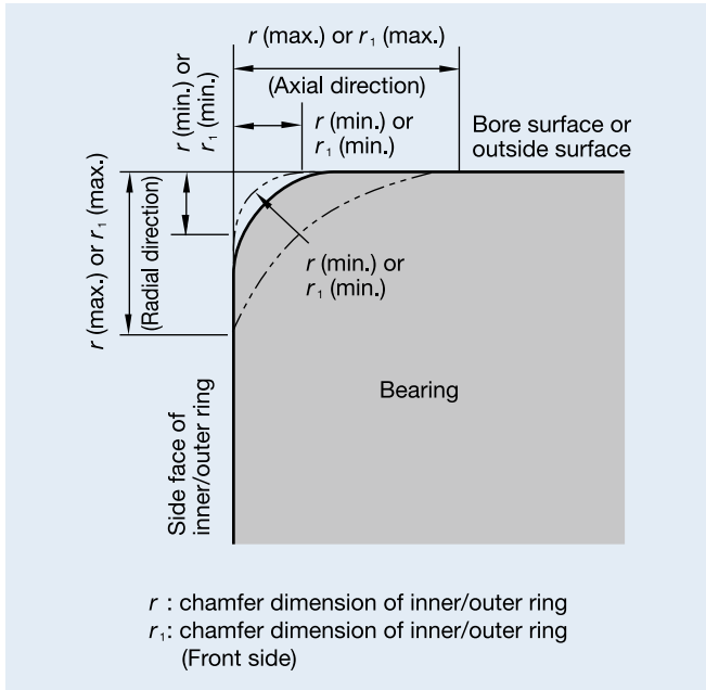
Fig. 8.2 Chamfer Dimension
